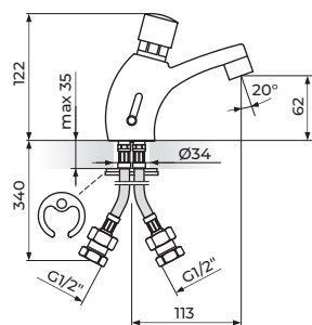
A73007 STOJEĆA BATERIJA TOPLA / HLADNA VODA
