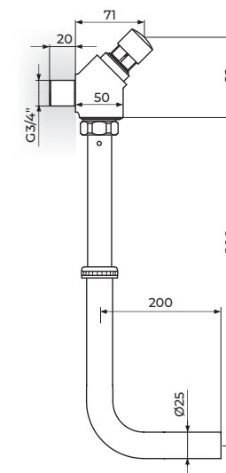
A79557 ISPIRAČ ZA WC MESINGANA PODESIVA CEV
